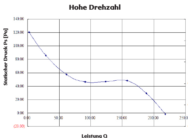
Strömungskennlinien, DV-PP-L-125 Lüfter
