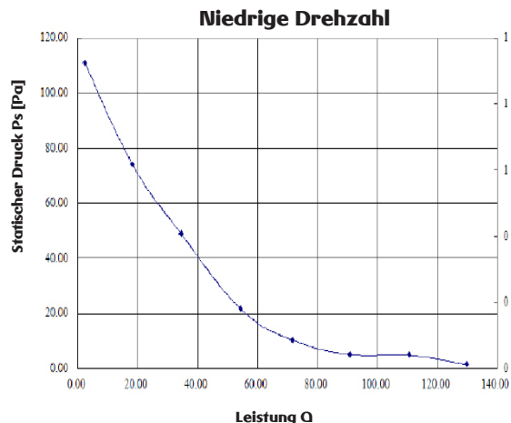
Strömungskennlinien, DV-PP-L-125 Lüfter
