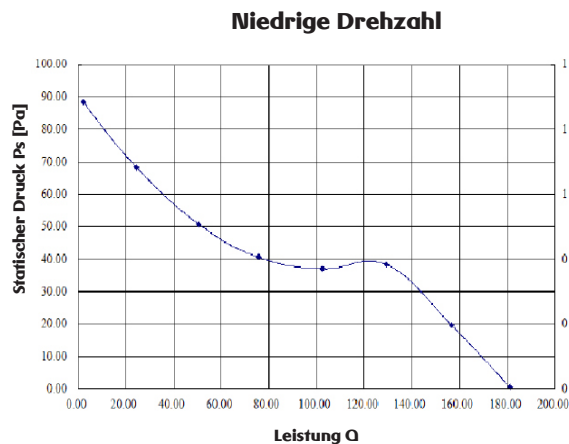
Strömungskennlinien, DV-PP-L-125 Lüfter
