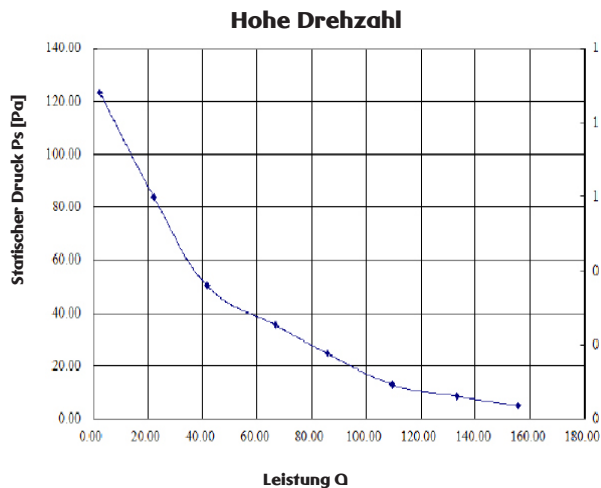
Strömungskennlinien, DV-PP-L-125 Lüfter
